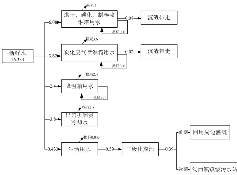
图 2-2 项目水平衡图（m 3 /d）
