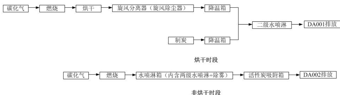
图 4-1 项目废气处理工艺流程图
