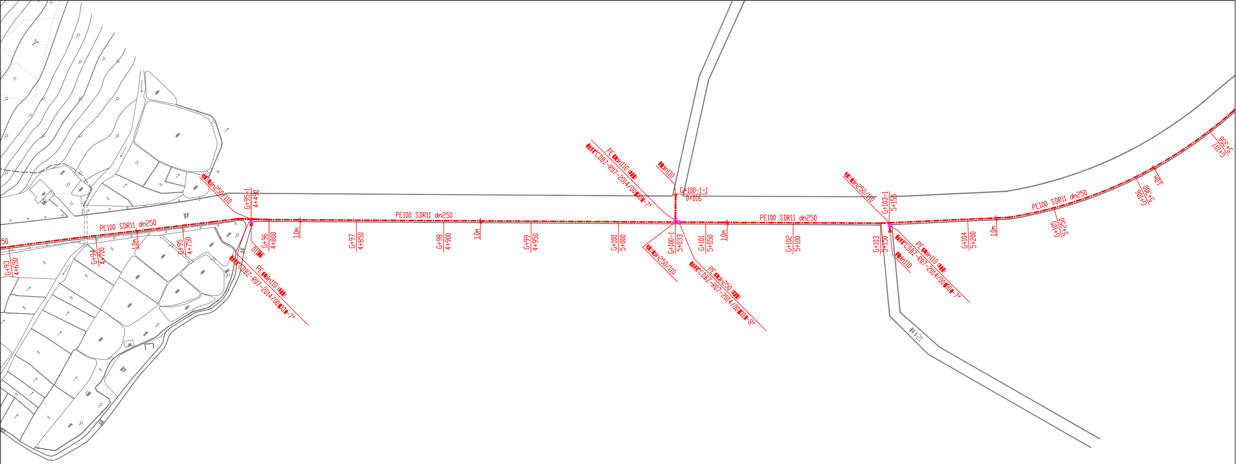
中压燃气管道平面布置图（八） 1:1000
