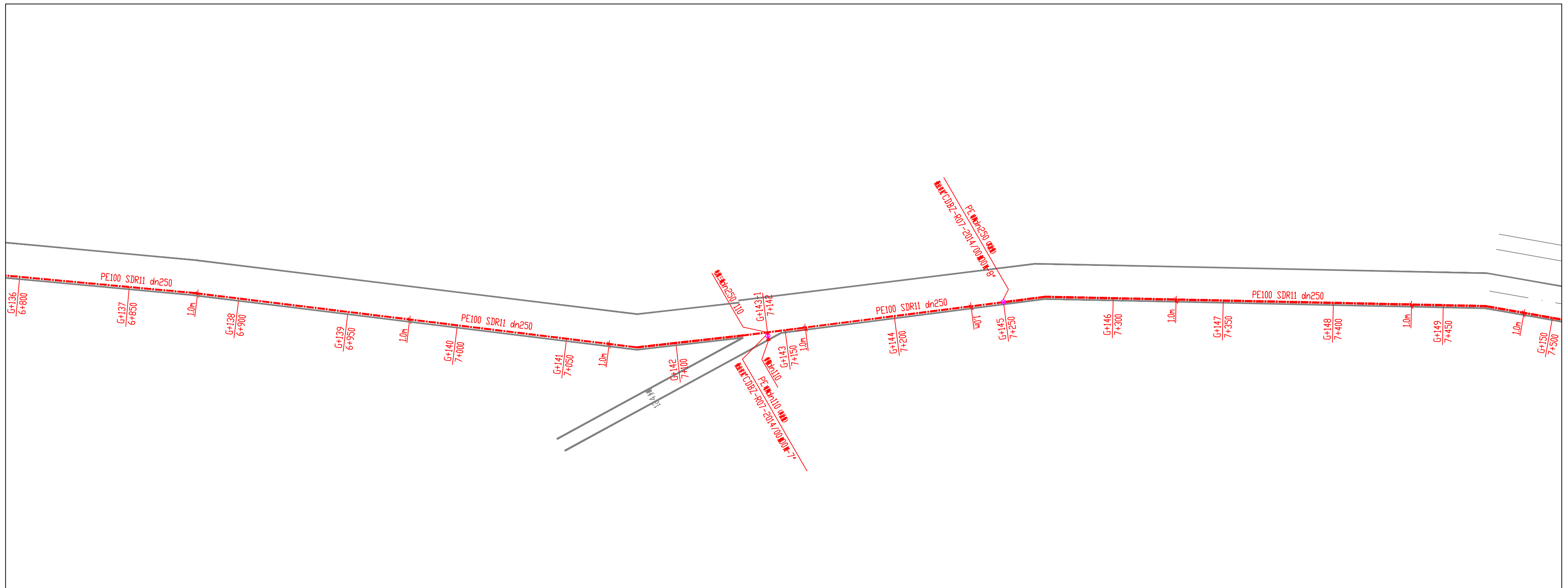
中压燃气管道平面布置图(十二) 1:1000
