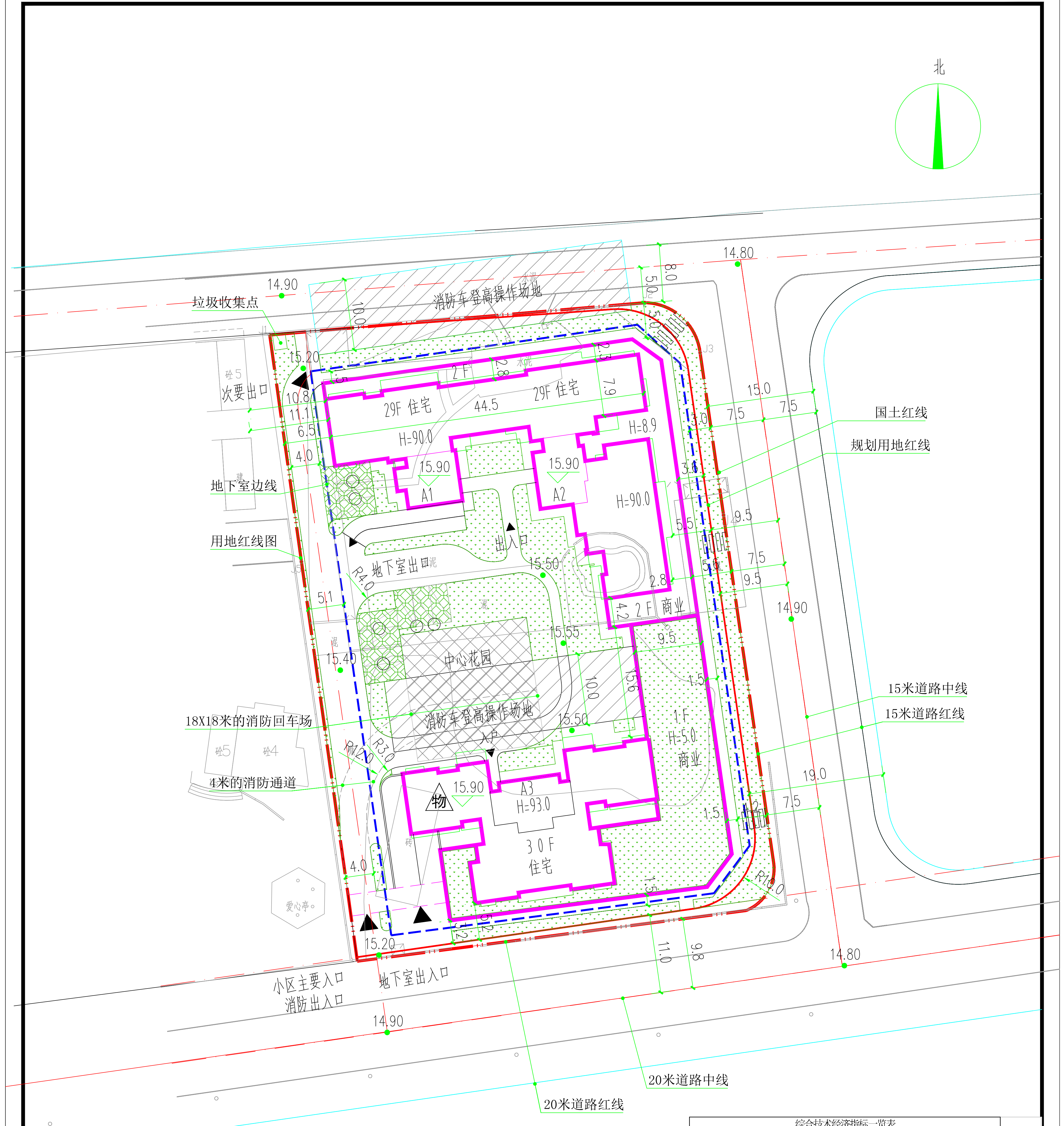
总平面图
